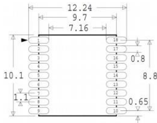
图 3- 1 ST310A模块封装尺寸示意图
