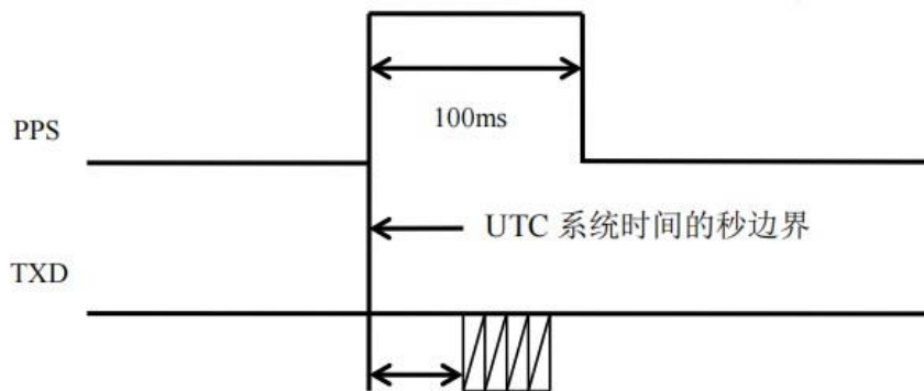
图 2-3 1PPS 秒脉冲示意图
