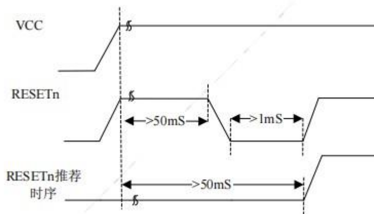
图 2-2 复位信号建议时序图
